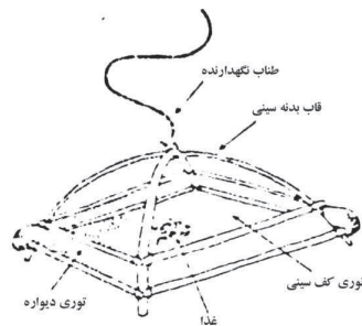
شکل ۱- ساختار و اجزاء سینی غذایی چهارگوشه (Cruz, 1991)
